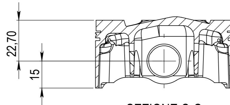
SEZIONE C-C
